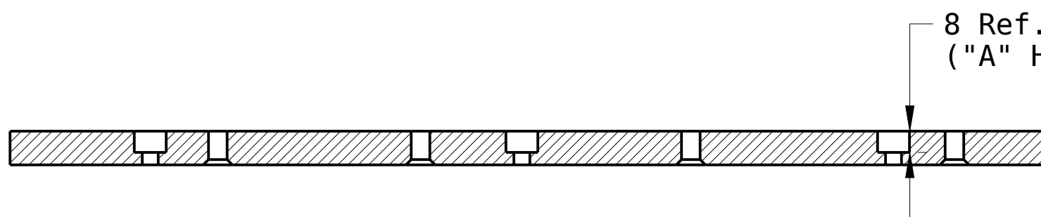
SECTION A-A
